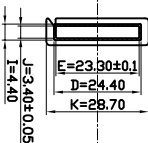
SECTION D-D
