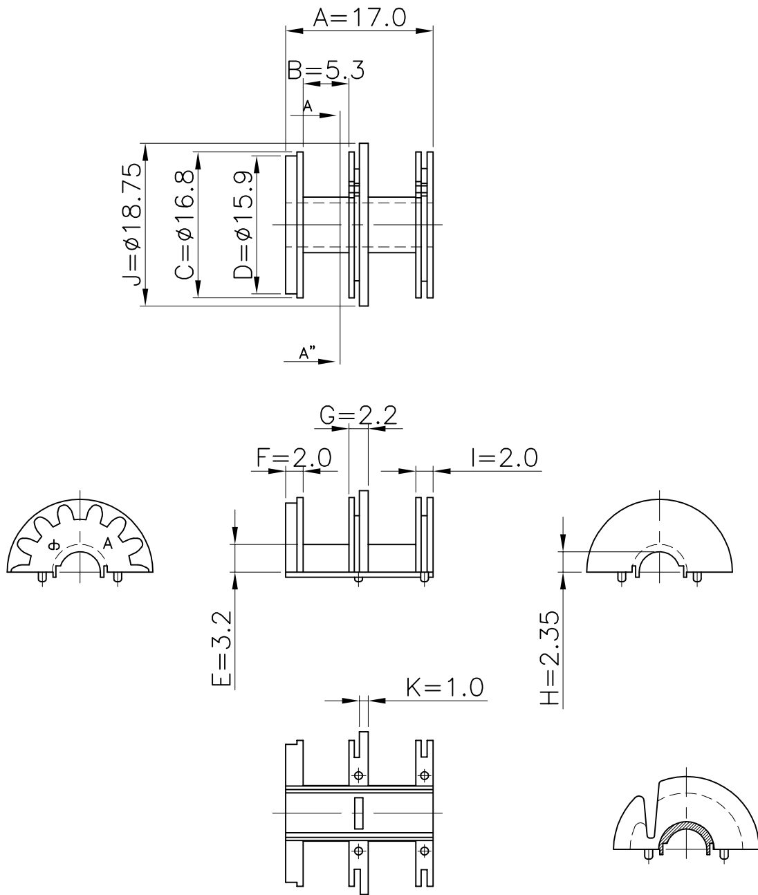
SECTION A-A
