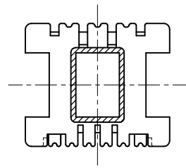
A-A SECTION
